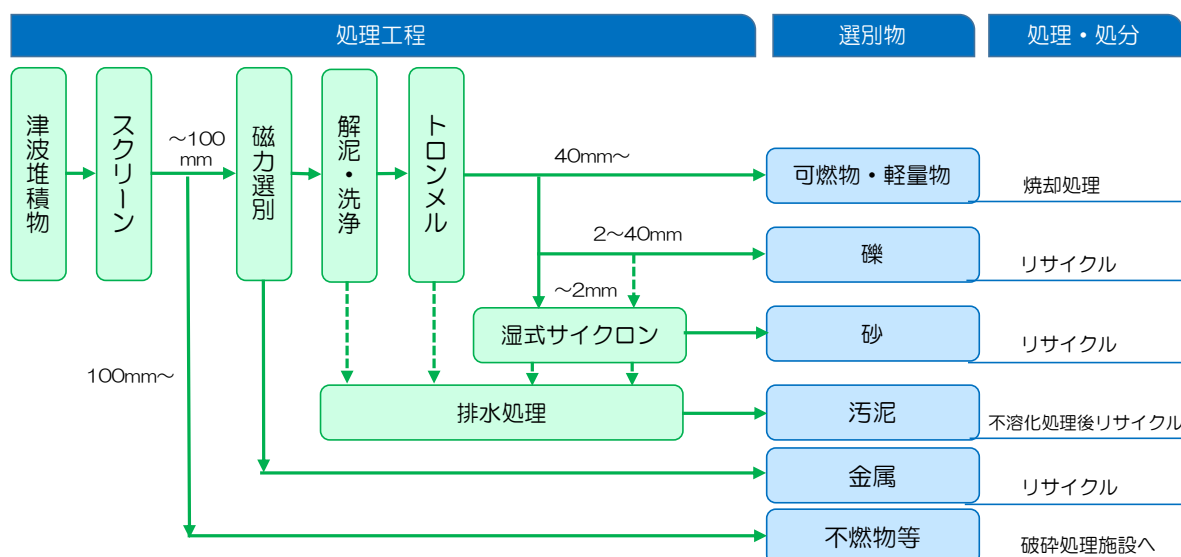
【湿式処理フローの例】
