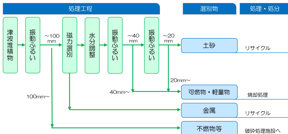
【乾式処理フローの例】
