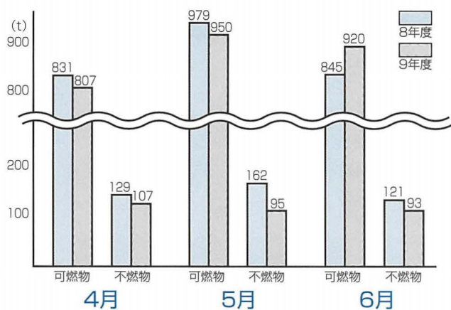
図2 資源ごみリサイクル実施前と後のごみ搬入量の推移
