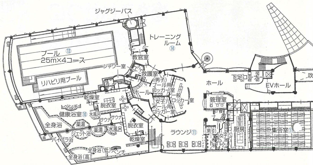
2階平面図
