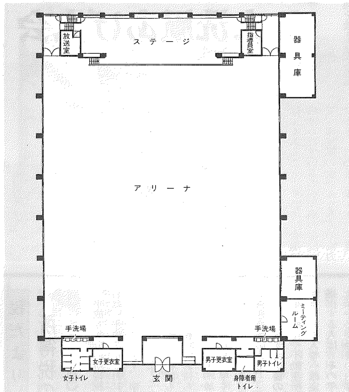
▲ 体育館（1階）平面図
