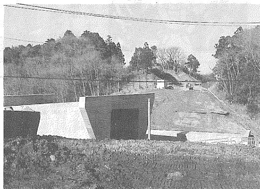
▲町道10号線と交差する隧道
