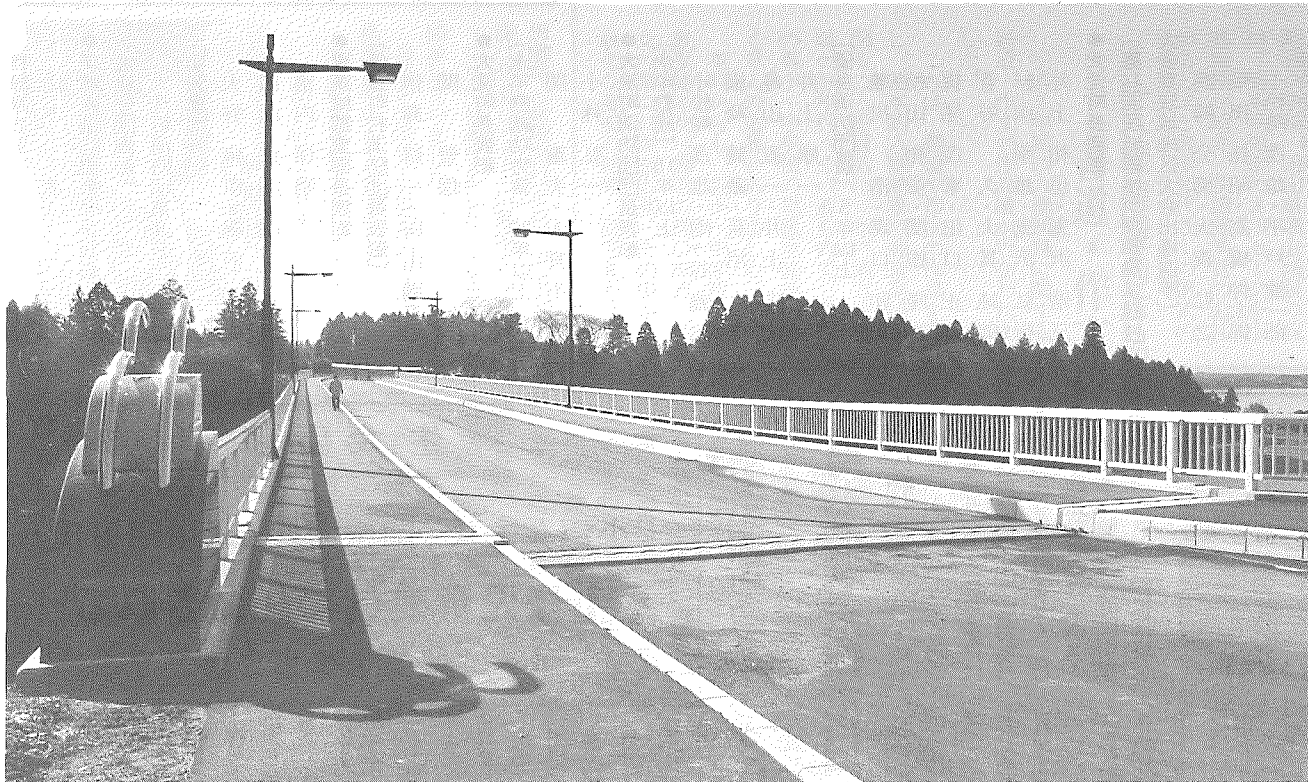
▲成田郷に架けられた成田高架橋
