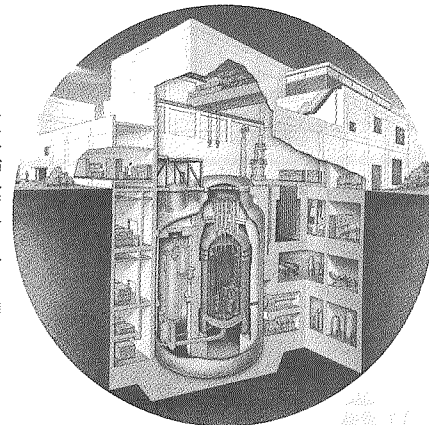
▶ 原子炉建家鳥かん図
