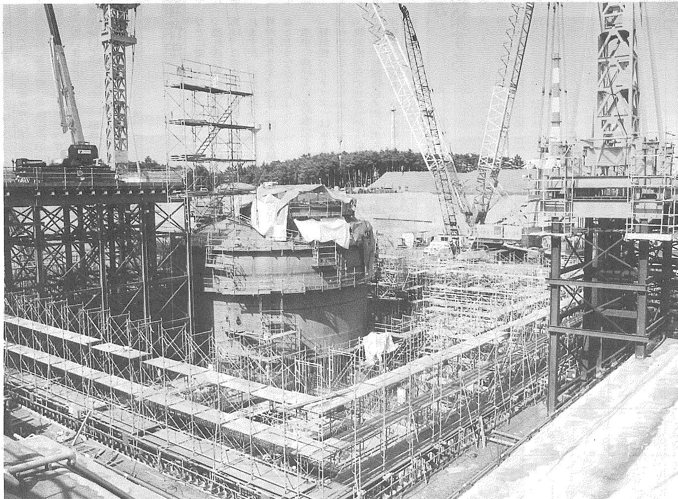
▲ 建設中の高温工学試験研究炉
