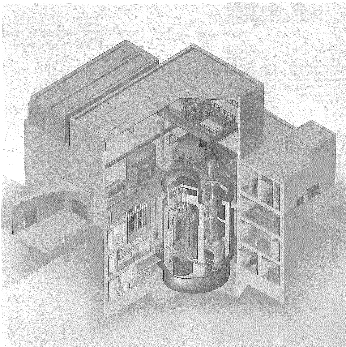
▲ 原子炉建家鳥かん図
