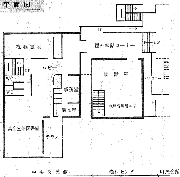
2階平面図
