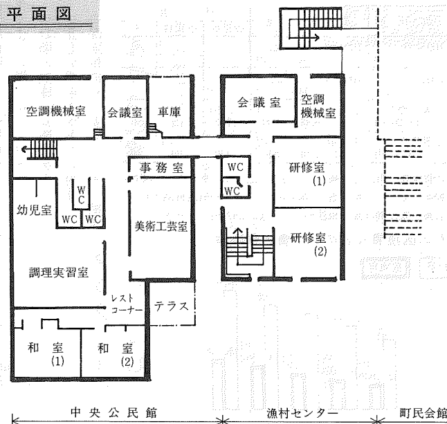
1階平面図
