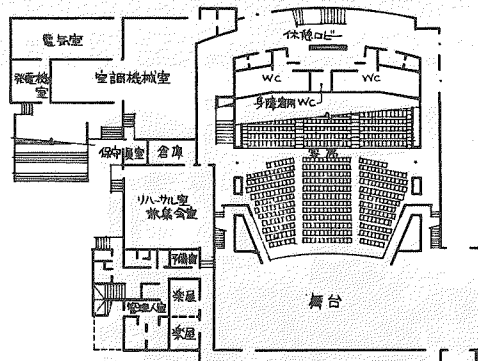
2階平面図
