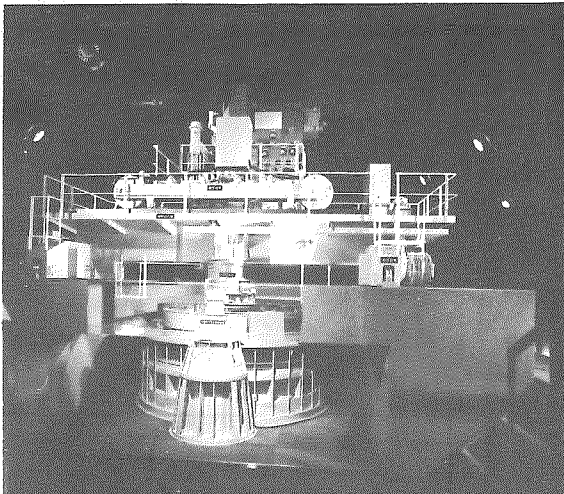
〈高速実験炉「常陽」上部機構〉
