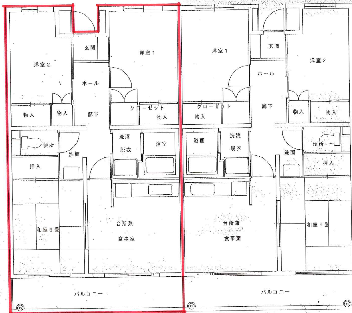
二葉住宅 C 棟平面図 65.34m 2
