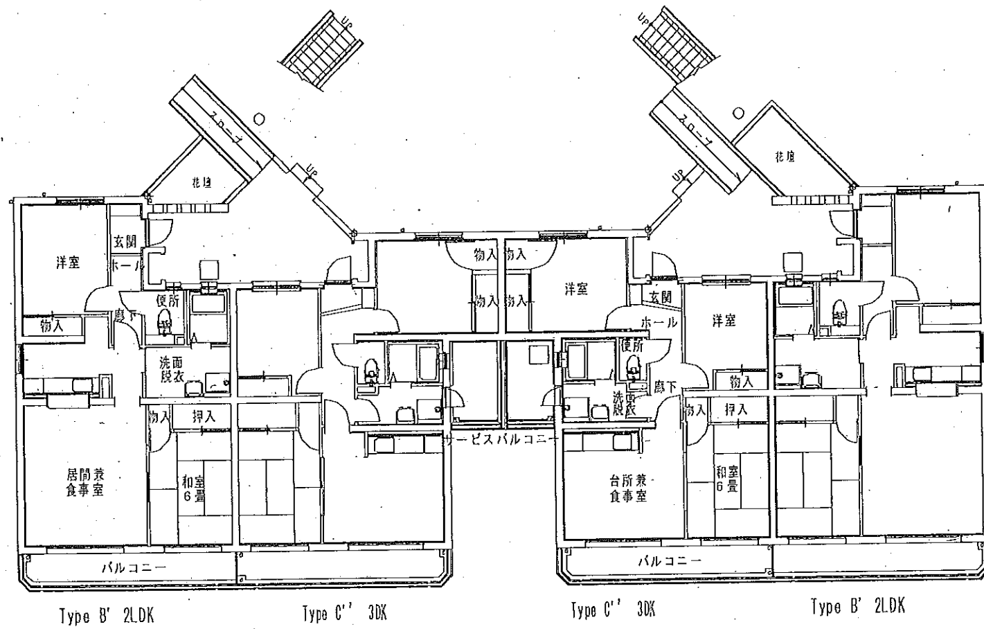
二葉住宅 D 棟平面図
