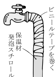
立上り管の保温方法
