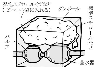
量水器の保温方法
