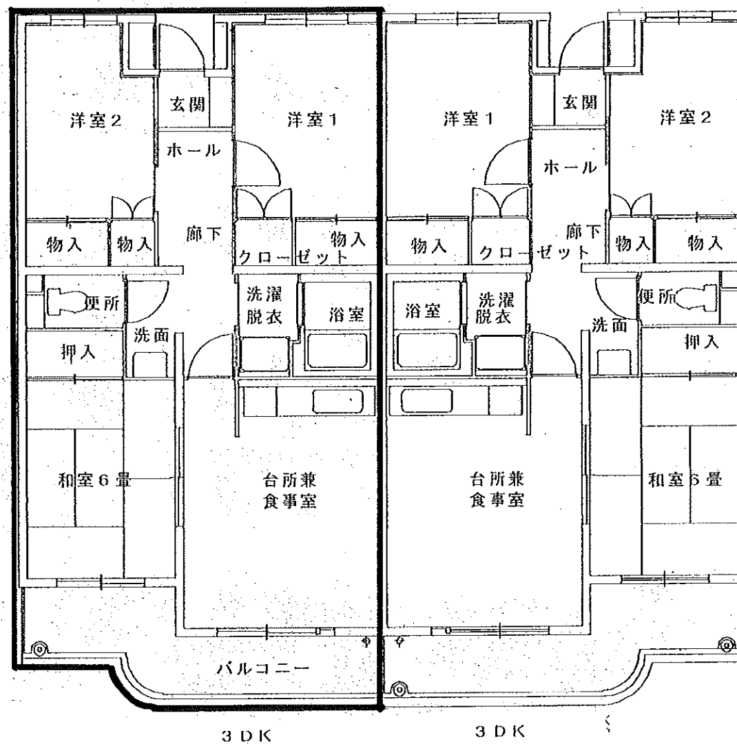
二葉住宅A棟平面図 68.67㎡
