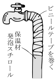
立上り管の保温方法
