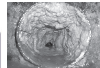
油脂類の堆積により閉塞した下水道管
