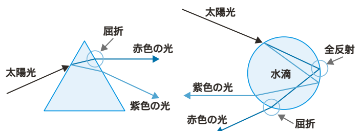
プリズムでの光の分解
